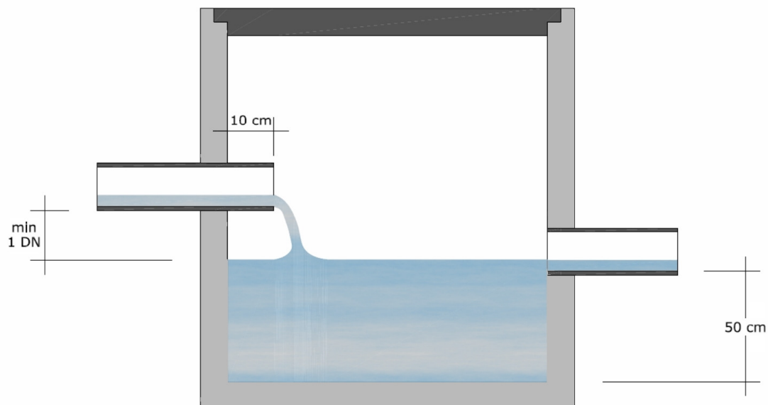
POZZETTO DI CAMPIONAMENTO
