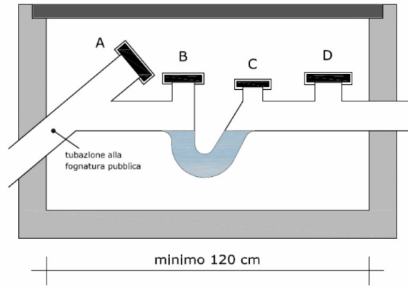
CAMERETTA DI ISPEZIONE TIPO BRAGA-SIFONE-ISPEZIONE (BSI)
